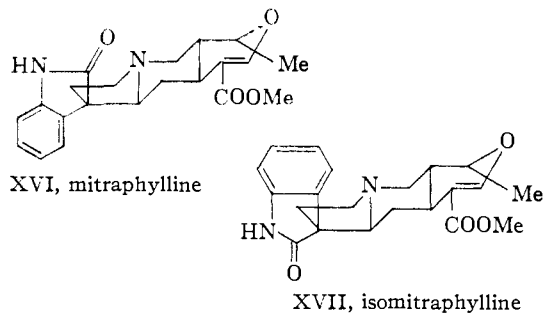
XVII, isomitraphylline
